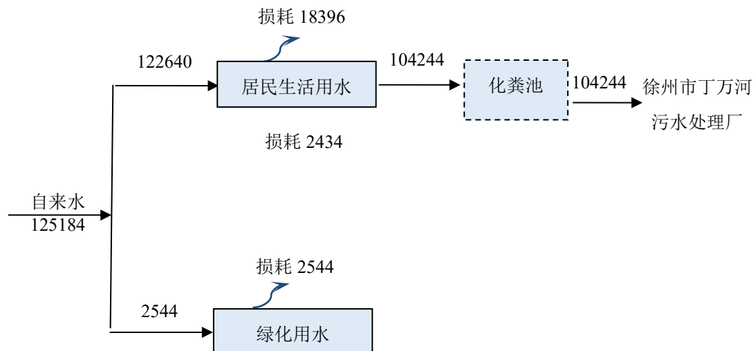
图 3-1 水平衡图（单位：m 3 /a）
